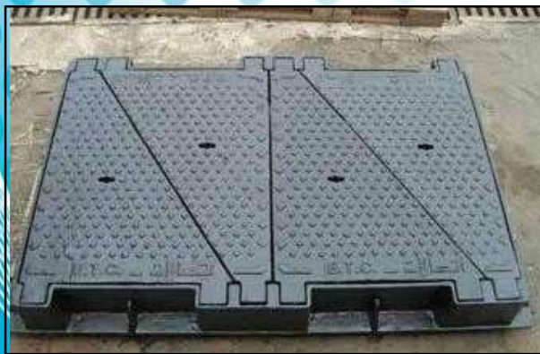
NẮP BỀ CÁP KT 155×884 TẢI 12,5T Model: NBC-155x884 / Tiêu chuẩn: BS EN124
